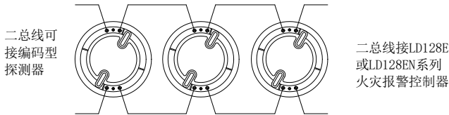
探测器及底座接线图
